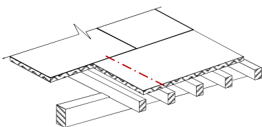
Recouper la dalle à l'axe de la solive
