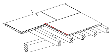
Vérifier que l'appui est suffisant
