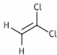
1,1-dichloro éthylène
