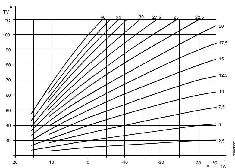
Diagramme de la caractéristique de chauffe
