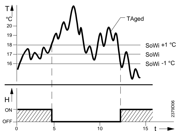
Commutation entre régime d'été et régime d'hiver
