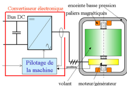
Fig. 4- Architecture générale d'un accumulateur à volant d'inertie
