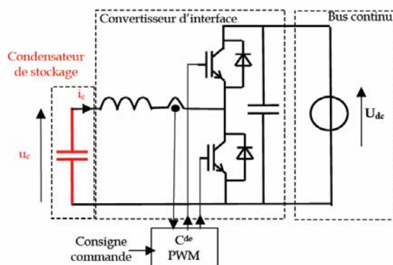
Fig. 3- Interface électronique de puissance entre un réservoir d'énergie capacitif et une source de tension continue (« bus continu »).
