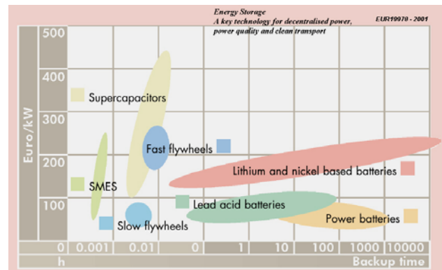
Fig. 7b- Coût de la puissance installée en fonction de la « constante de temps » (source : [CEE_01])
