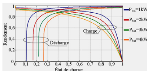
Rendement global en charge et en décharge, en fonction de l'état de charge et paramétré en puissance
