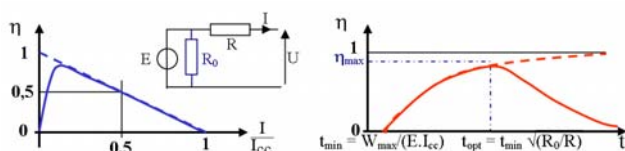
Fig. 2- Schéma électrique de principe permettant de mettre en évidence l'effet du courant ou du temps de décharge sur le rendement ( W_{\text{max}} = E \cdot Q ). Les courbes en pointillés correspondent à un modèle sans résistance d'autodécharge.
