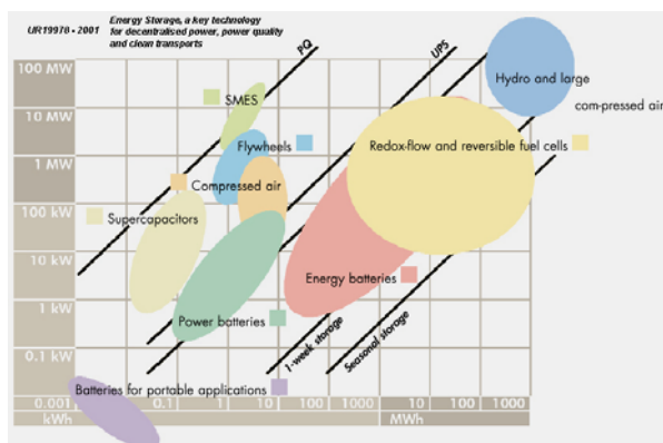
Fig. 7a- Domaines d'applications en puissance et énergie de technologies de stockage en applications réseaux ([CEE_01])
