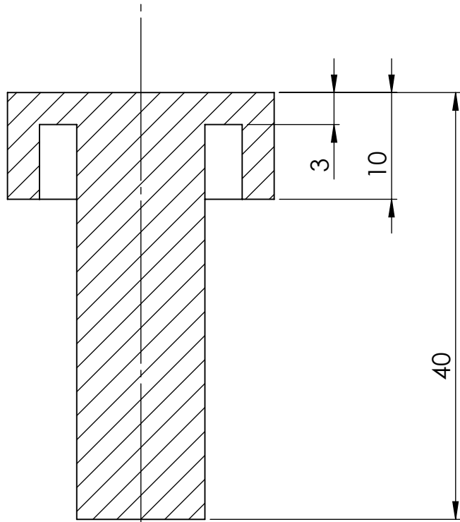
COUPE A-A
