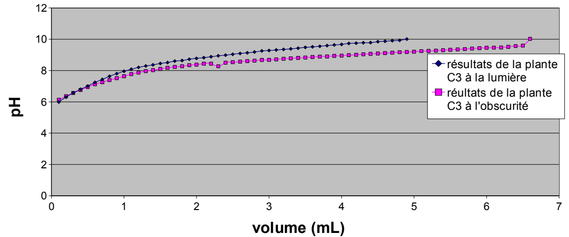
Courbe représentant le pH en fonction du volume de NaOH
