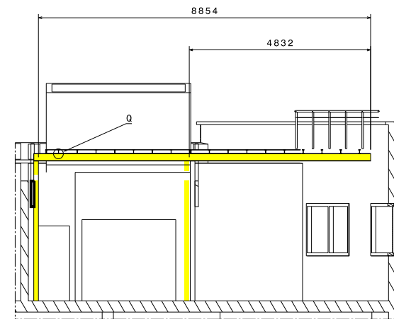
Coupe J-J[2] Echelle : 1:50
