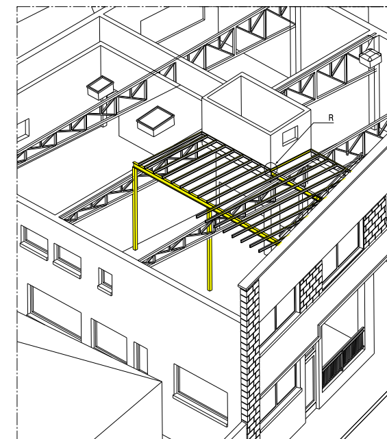
Vue isométrique[3] Echelle : 1:70
