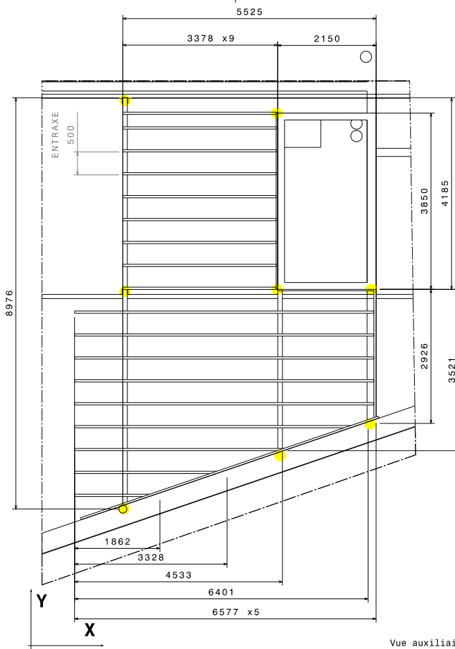
Vue auxiliaire O Echelle : 1:40
