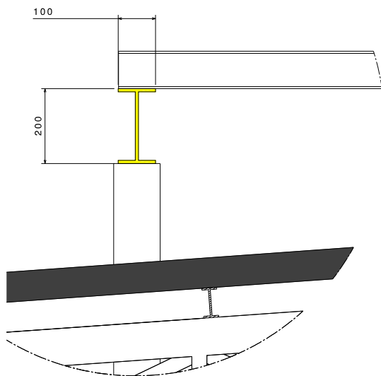
Détail P Echelle : 1:5
