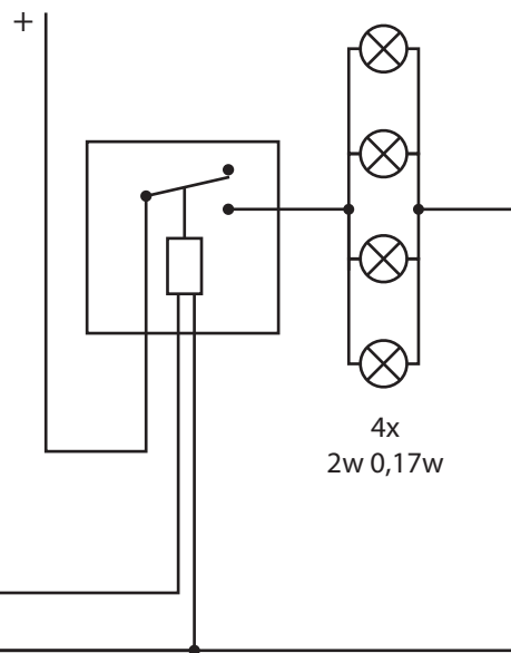
Circuit secondaire
