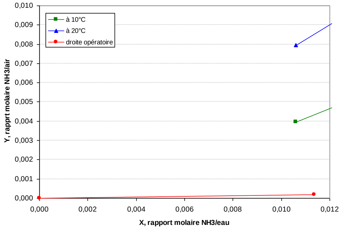
Courbe d'équilibre eau-NH3-air
