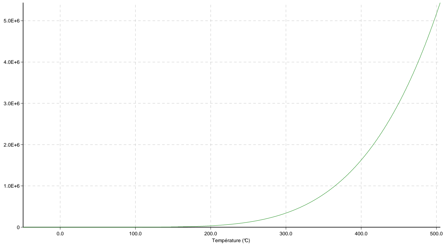
Pression de vapeur saturante (Pa) - Formulation N° 101
