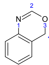
4H-3,1-benzoxazine
