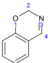
2H-1,3-benzoxazine
