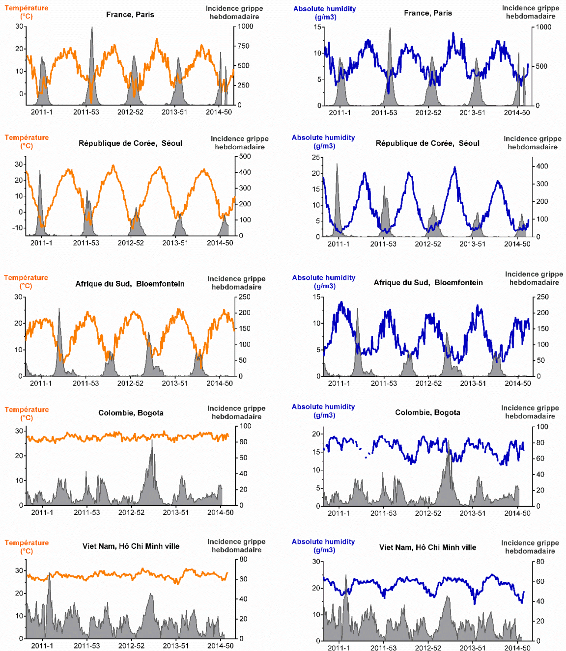
Figure I-13 : Suivi de l'incidence hebdomadaire des virus grippaux de type A dans différents pays et sur 5 années, en fonction du climat local. La France, la République de Corée et l'Afrique du Sud sont des pays tempérés dans lesquels une forte saisonnalité des virus grippaux est observée. La Colombie et le Viêt Nam sont des pays au climat tropical, marqués par une transmission à bas bruit des virus grippaux tout au long de l'année. Les données épidémiologiques (surfaces grises) ont été importées de la base de données FluNet, mise en place par l'Organisation Mondiale de la Santé. Les données météorologiques ont été récupérées à partir du site internet participatif de données météorologiques www.wunderground.com . L'axe des abscisses représente les Années-semaines.
