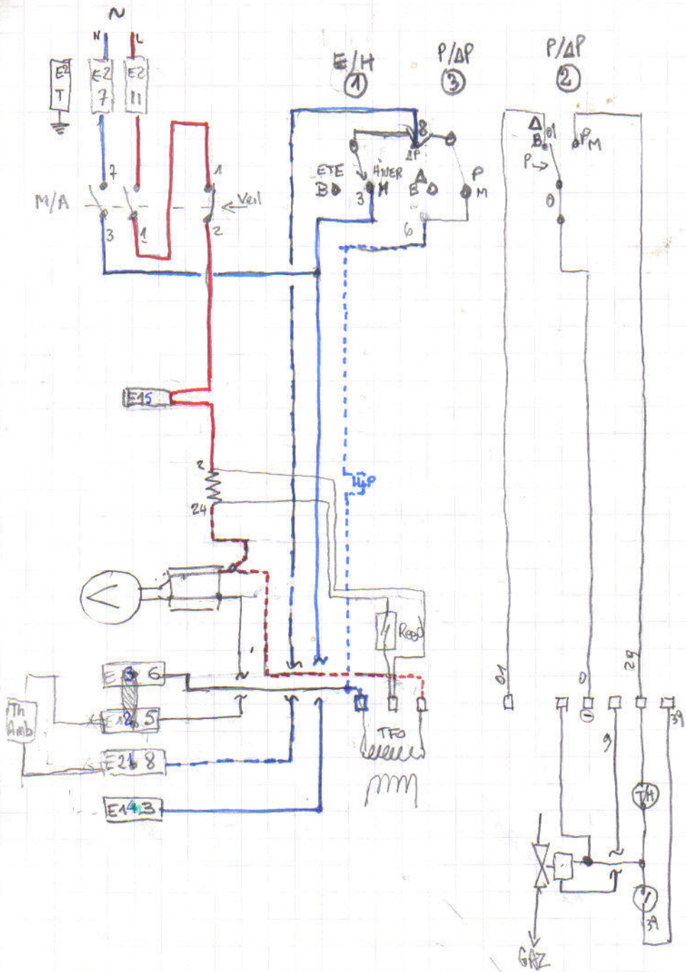
SCHEMA CHAUDIERE
