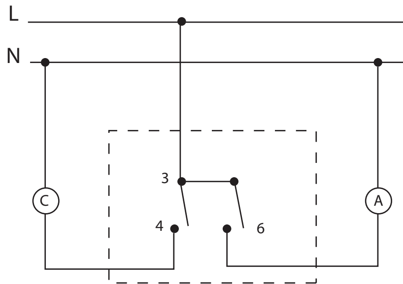
Schéma constructeur du thermostat
