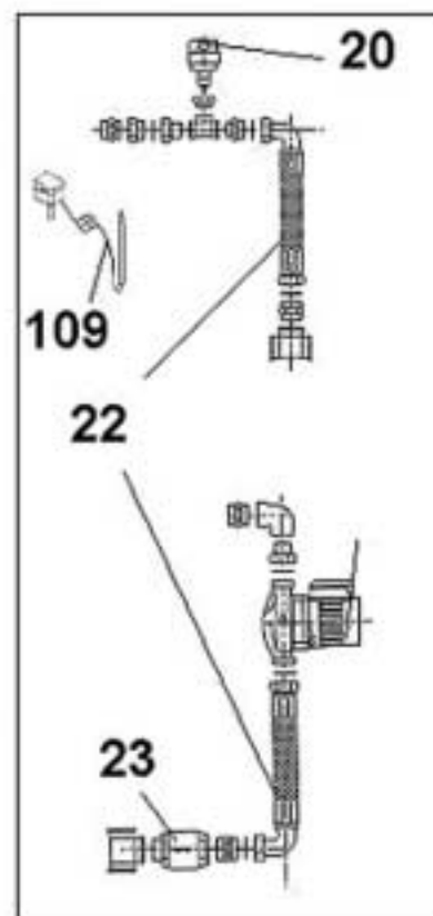
Kit pompe pour tous modèles
