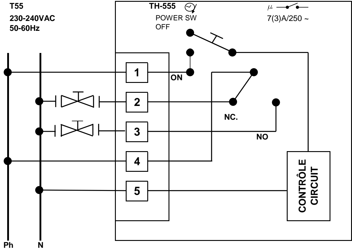
SCHÉMA SE TROUVANT DANS LE COUVERCLE
