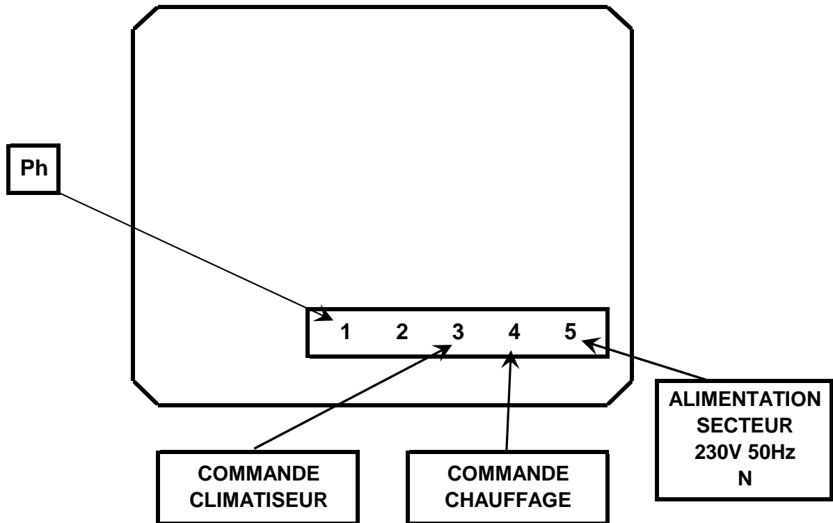
SCHÉMA SE TROUVANT SUR LA NOTICE
