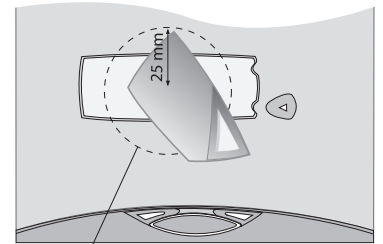
Le badge est détecté dans cette zone à une distance d'approche de 20 mm maximum
