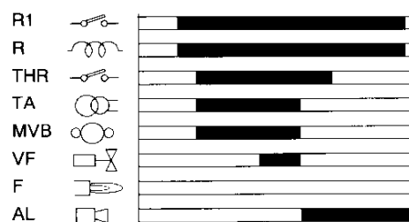
Diagramme de mise en sécurité Sans apparition de flamme
