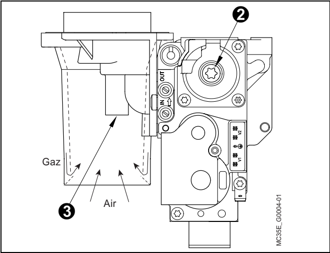
2 Vis Torx : Correction du pourcentage O 2 /CO 2 en petite allure
