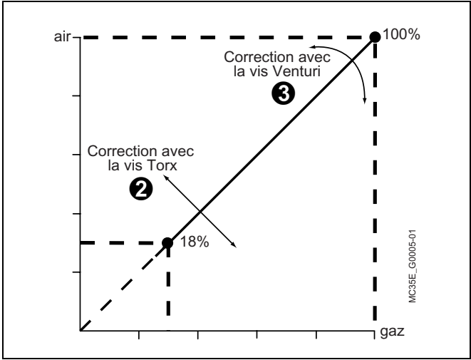
3 Vis Venturi : Correction du pourcentage O 2 /CO 2 en grande allure
