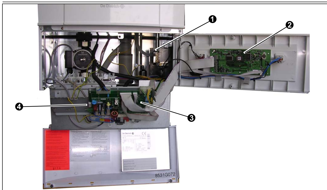
Platine carte en position d'entretien
