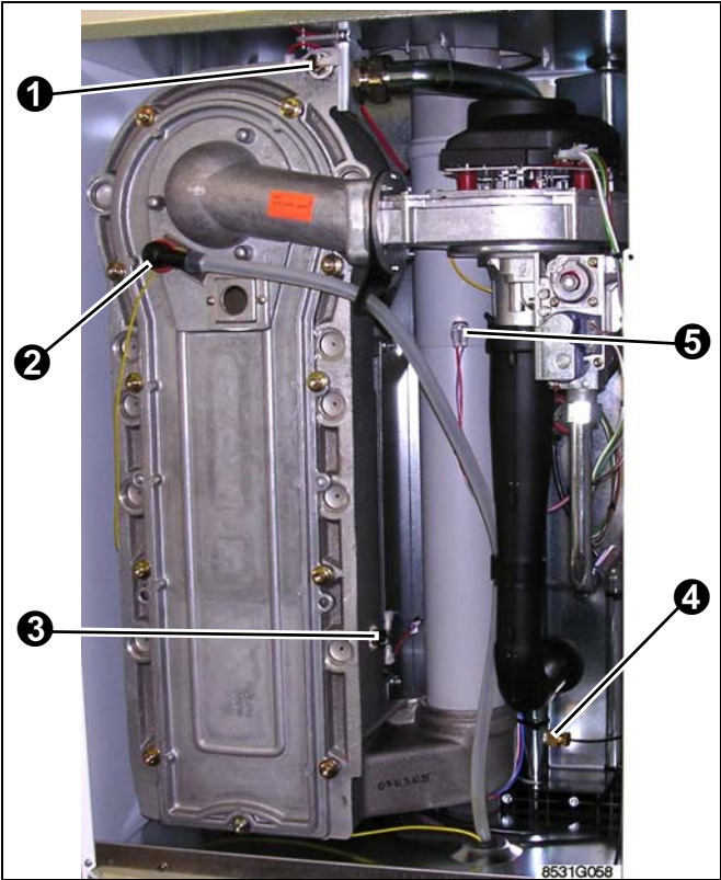
MC 35E, MC 45 et MC 65
