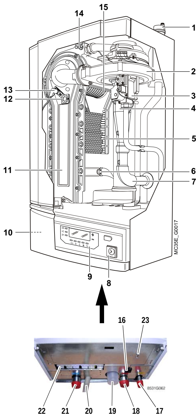
Exemple du modèle MC 35E
