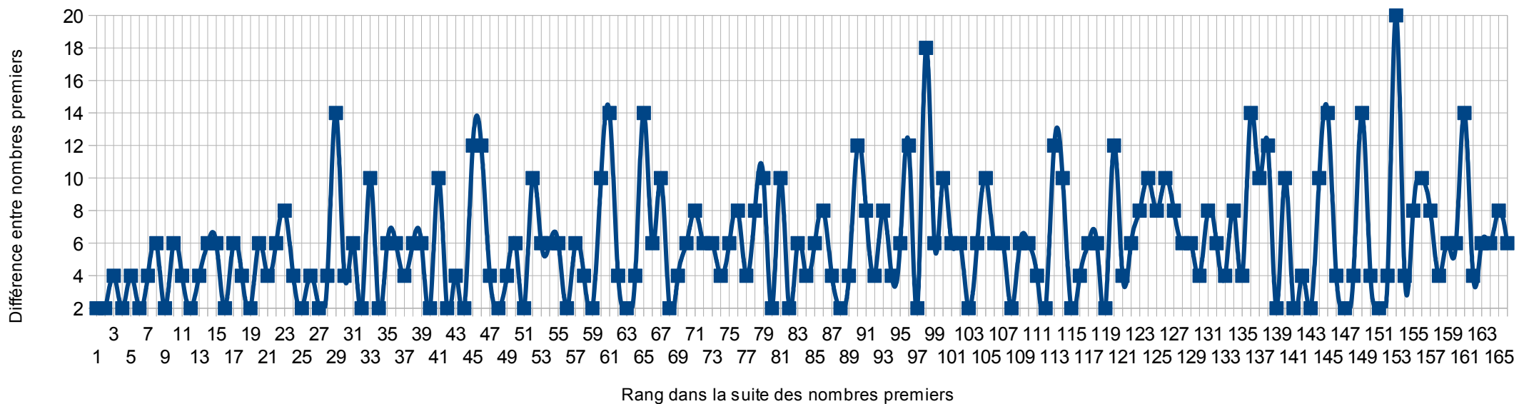
Variation de la différence entre nombres premiers en fonctions de leur rang dans la suite
