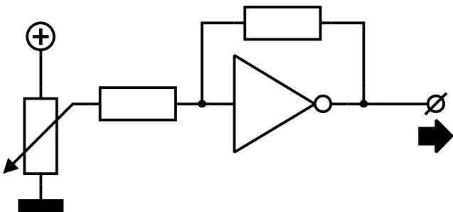
Buffer pour potentiomètre
