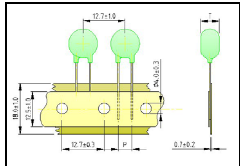
Ammo Taping Type
