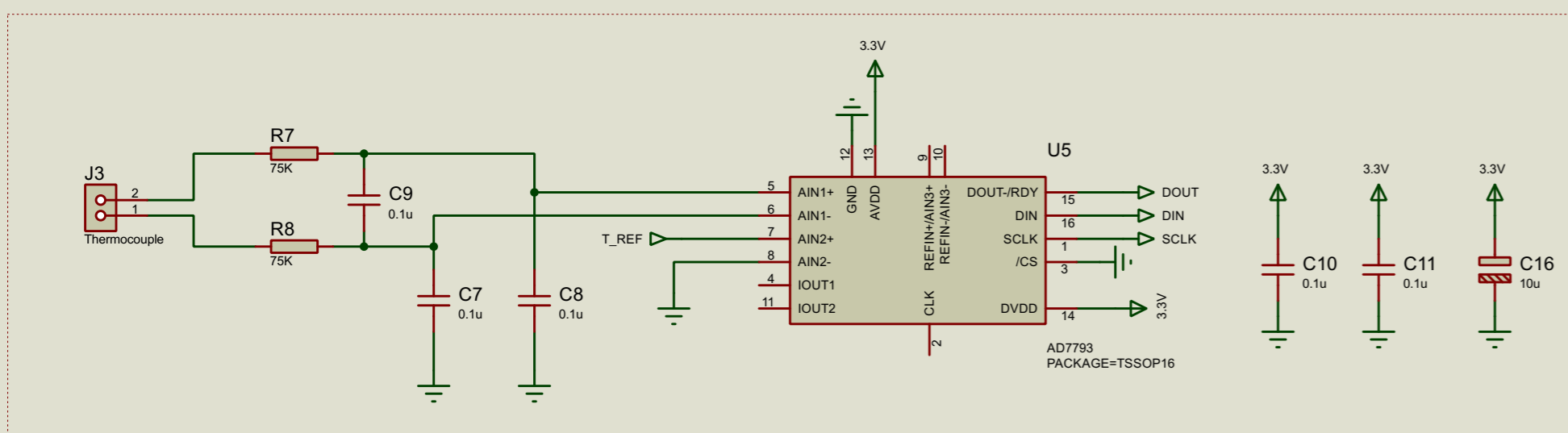
Mesure thermocouple
