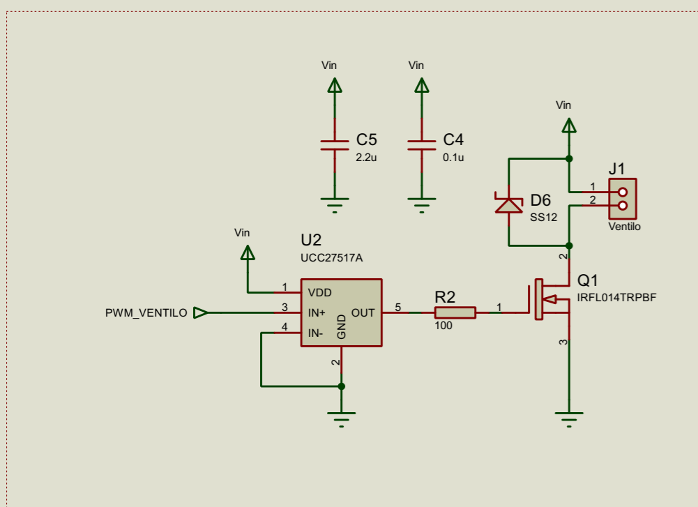
Controle ventilo partie commande
