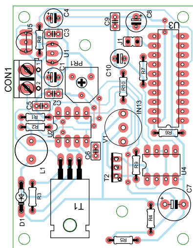
Rysunek 3. Schemat montażowy termometru z lampą Nixie
