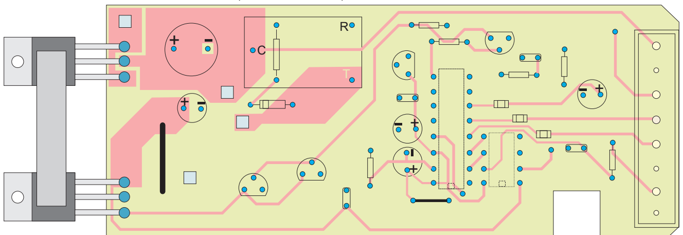
(VUE DE DESSUS) CUIVRE COUCHE SUPÉRIEURE
