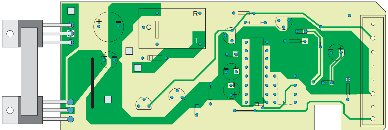
(VUE DE DESSUS) CUIVRE COUCHE INFÉRIEURE
