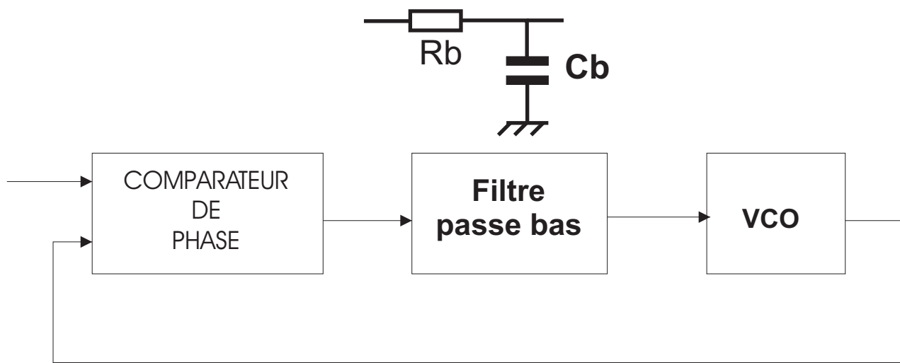
Principe du PLL
