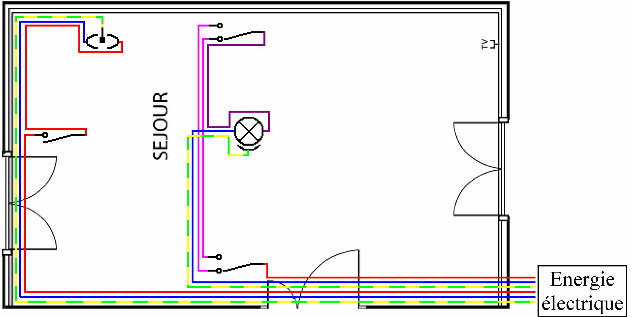
Schéma multifilaire
