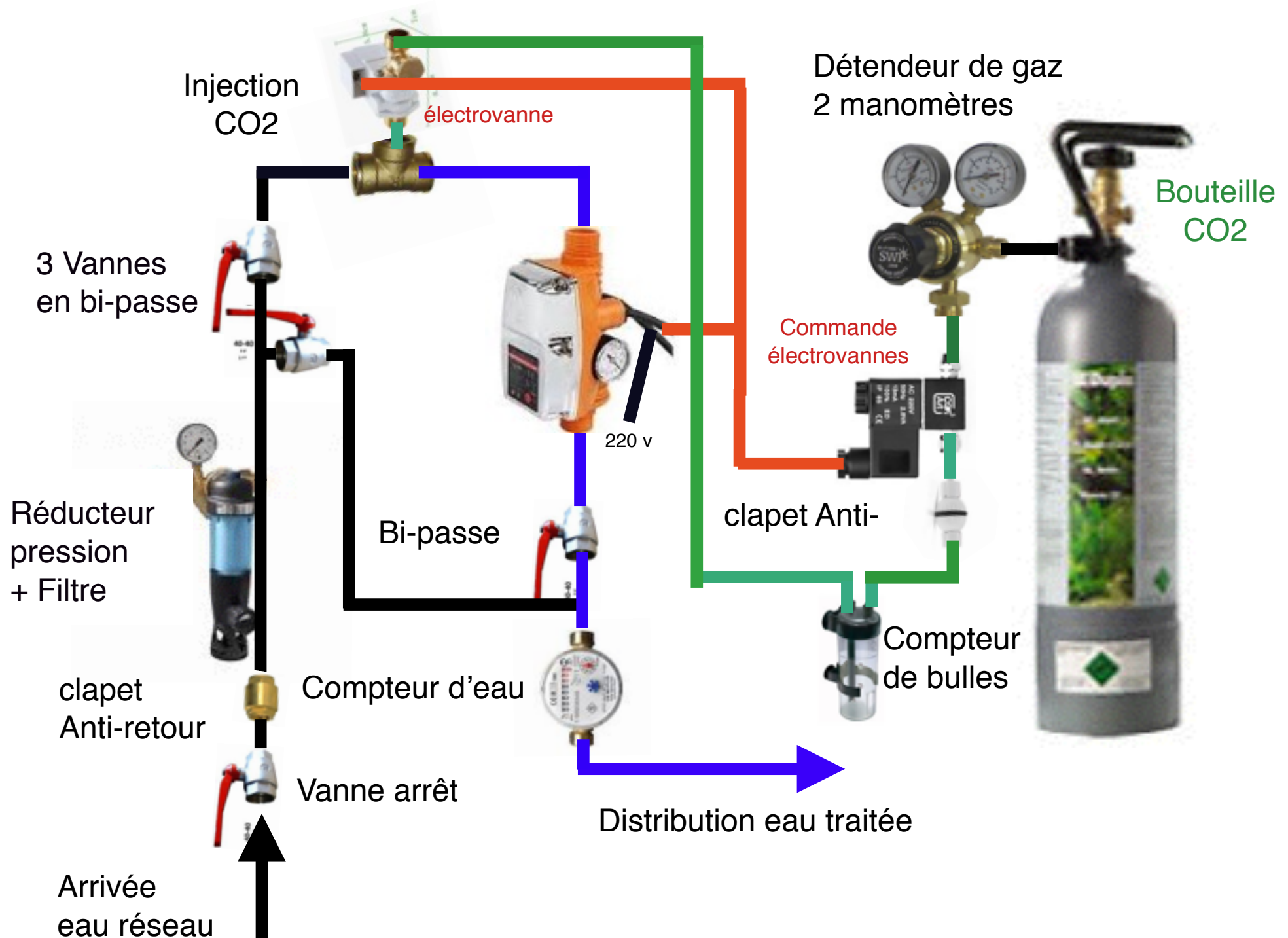
Shéma d'installation de traitement de l'eau par injection de CO2
