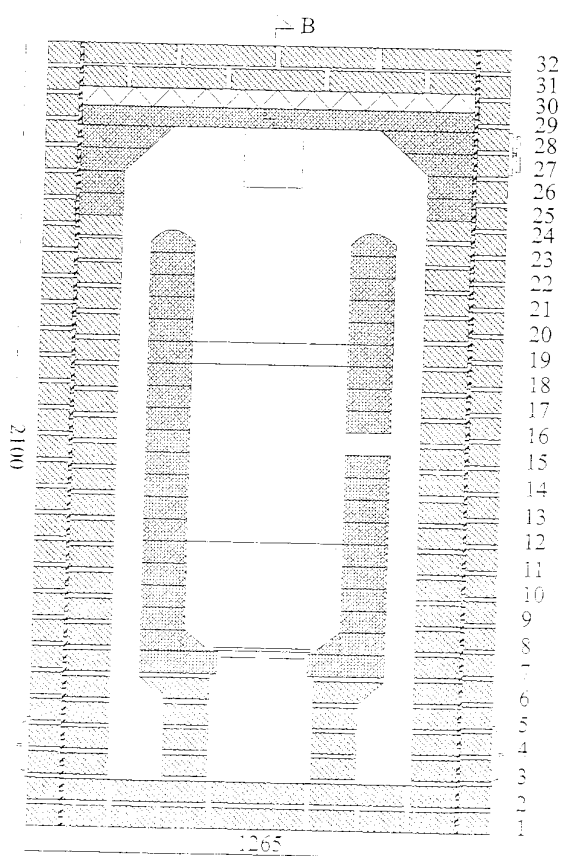
Leikkaus A
