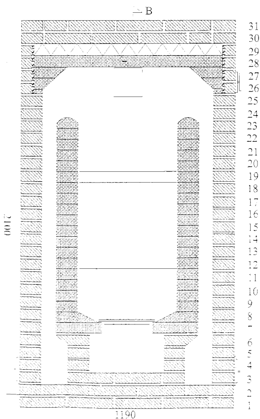
Leikkaus A
