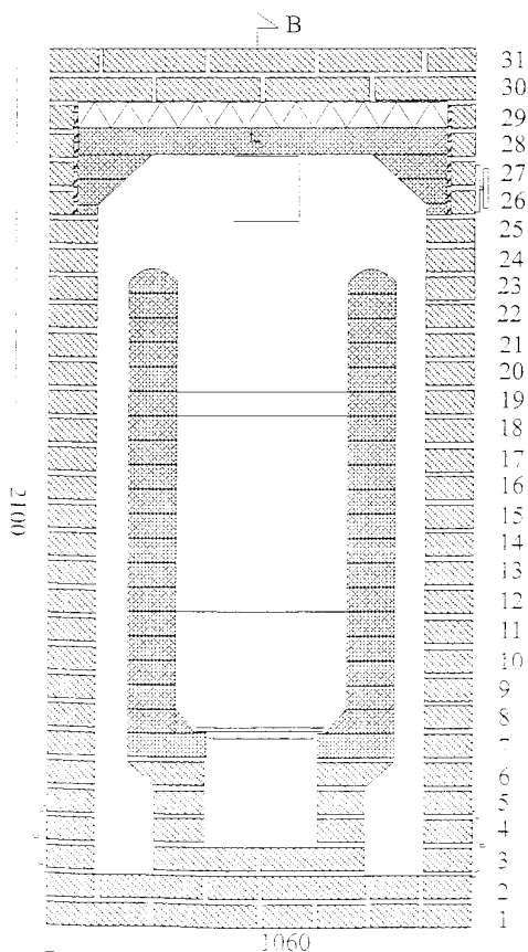
Leikkaus A
