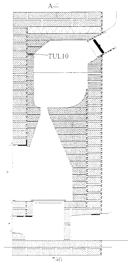
Leikkaus B
