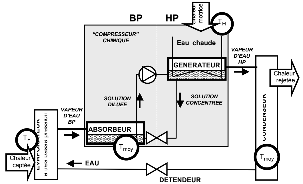
Pompe à chaleur chimique
