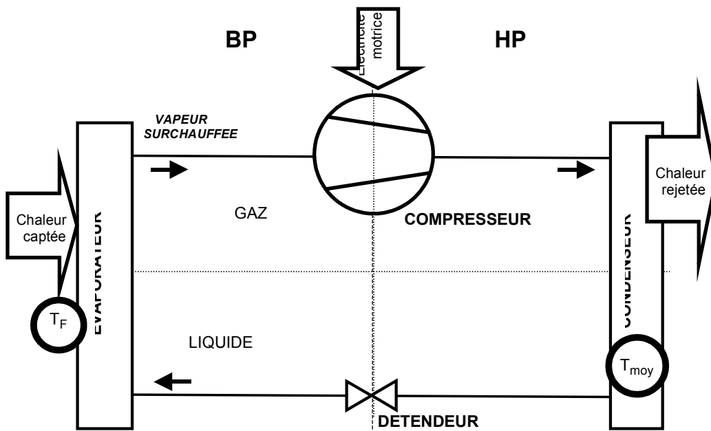
Pompe à chaleur électrique
