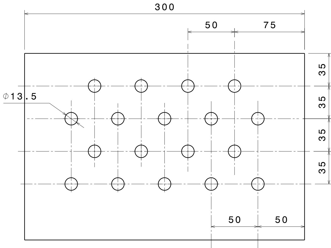
Vue de face Echelle : 1:2
