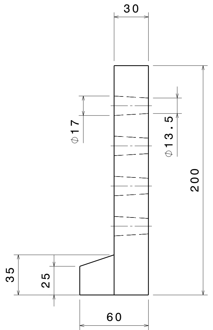
Vue de gauche Echelle : 1:2
