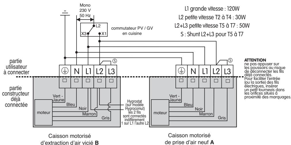
Schéma de câblage des ventilateurs
