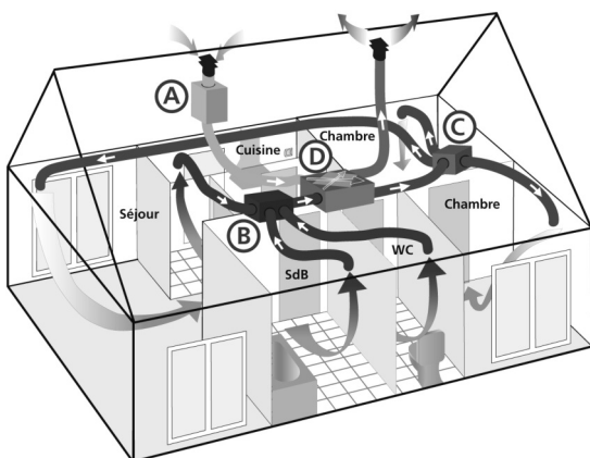
Caisson motorisé de prise d'air neuf
