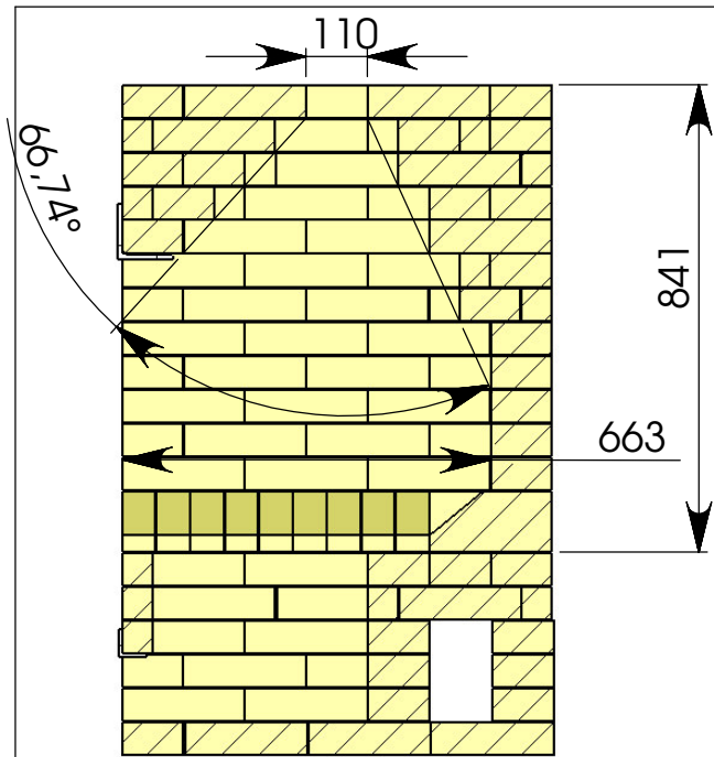
COUPE A-A
