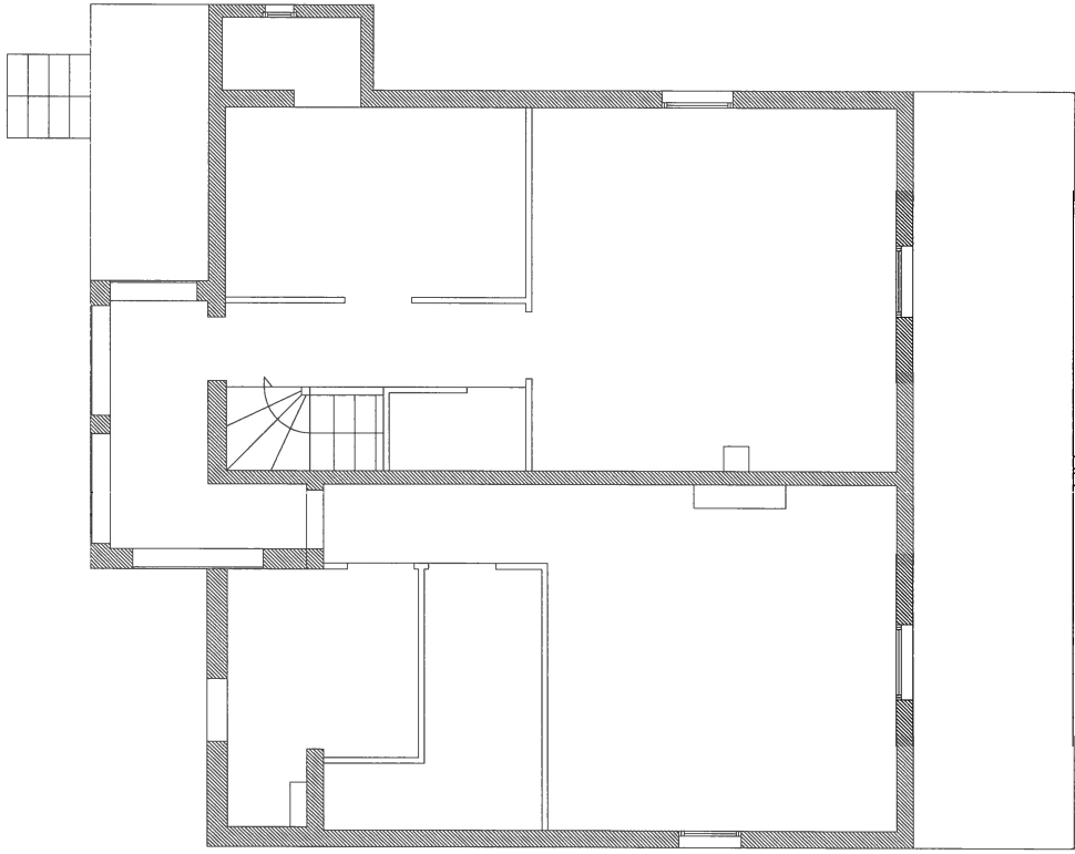
EDL - Etage - 1/100
