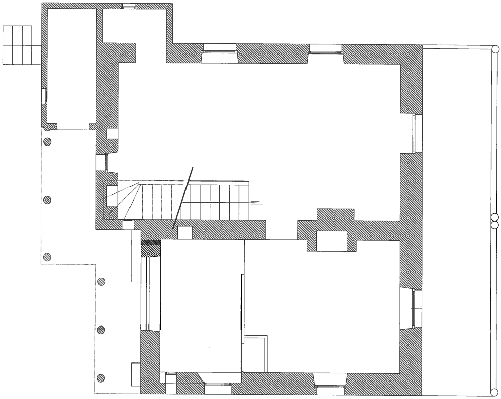
EDL - Rez de Chaussée - 1/100
