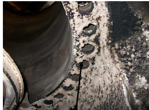
Partie inférieure de l'échangeur
