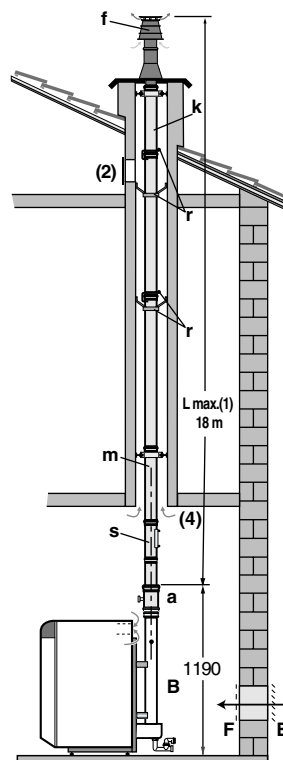
Raccordement sous le conduit de cheminée
