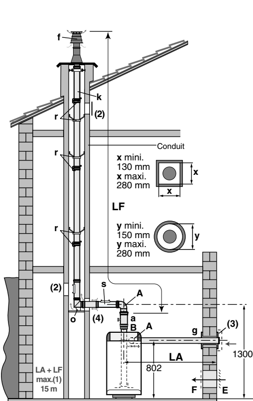
Raccordement perpendiculaire au conduit de cheminée
