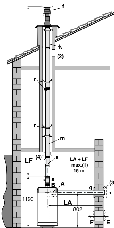
Raccordement sous le conduit de cheminée
