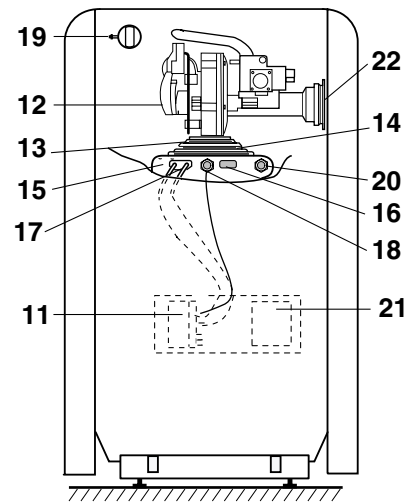
Vue de face / coupe
