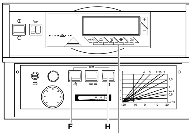
Sélection mode de fonctionnement (4)
