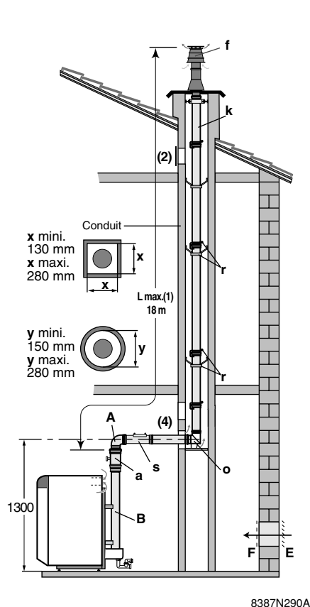
Raccordement perpendiculaire au conduit de cheminée
