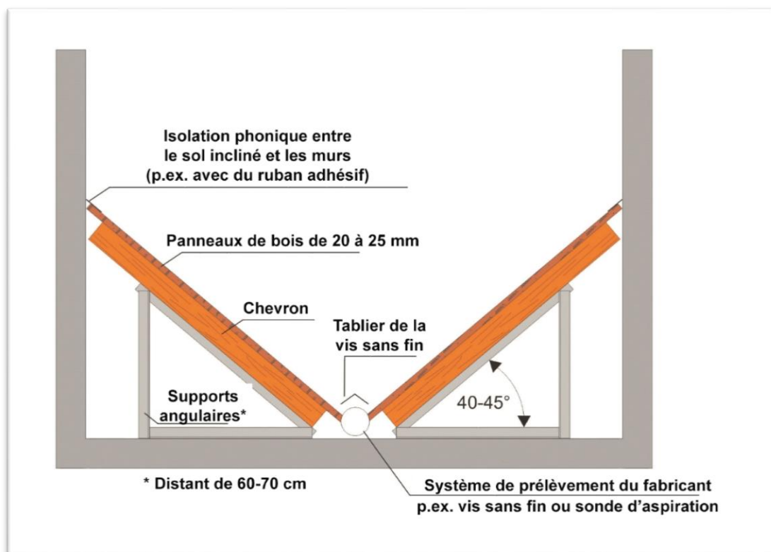
Figure 5 : Recommandations relatives à l'installation d'un silo à pans inclinés
