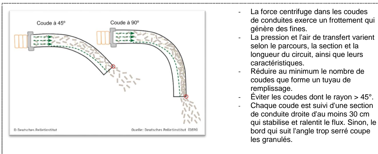
Figure 8 : Schéma de déchargement des granulés en fonction des coudes, sans section droite appropriée (section de ralentissement)
