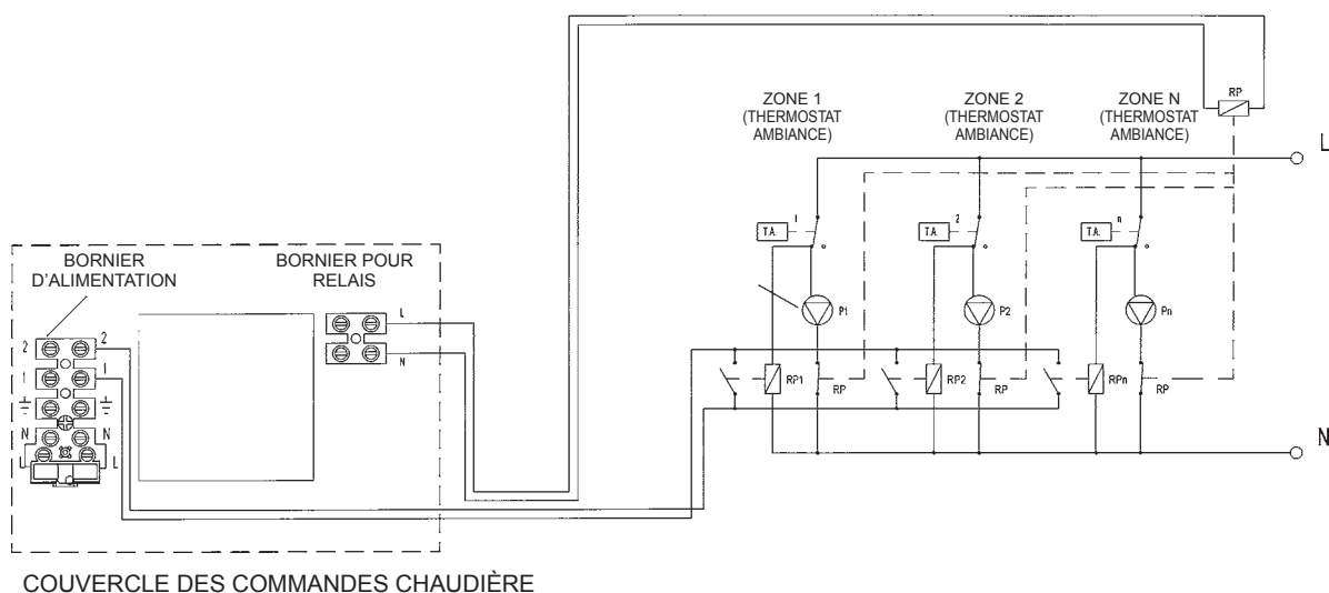
Figure 4: Schémas électriques de branchement des thermostats ambiance de zone et alimentation des pompes ou des vannes
