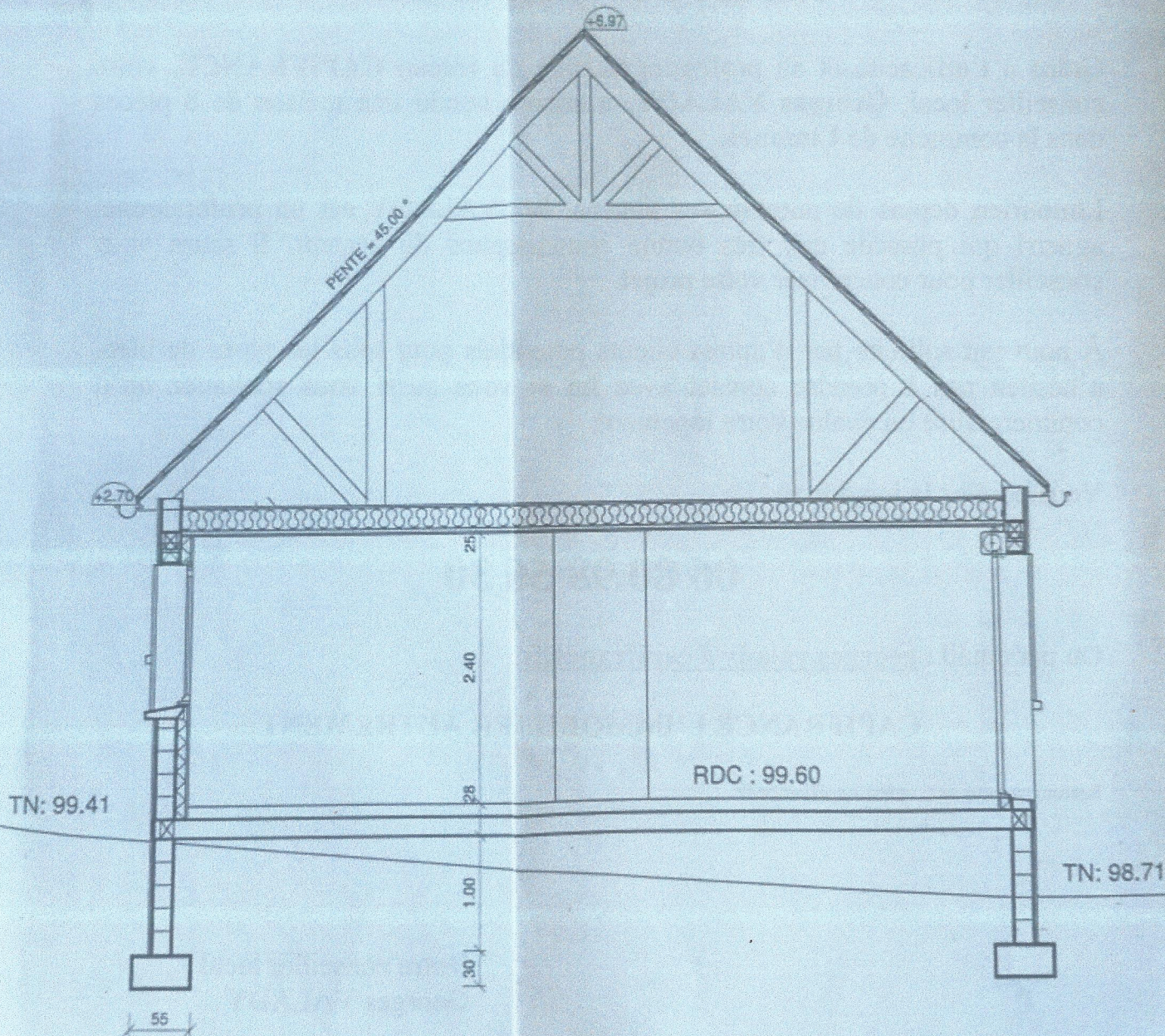
Coupe AA
