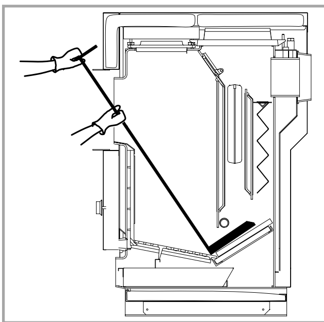
Figure 16 - Décrassage de la brique réfractaire
