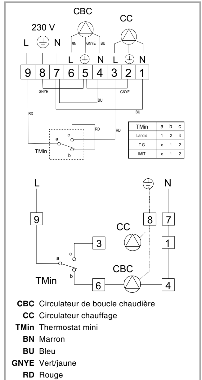
Fig. 10 - Câblage et schéma électriques
