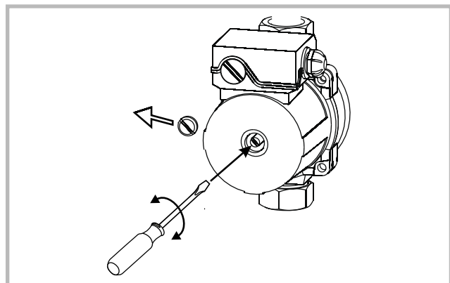
Figure 11 - Dégrippage du circulateur
