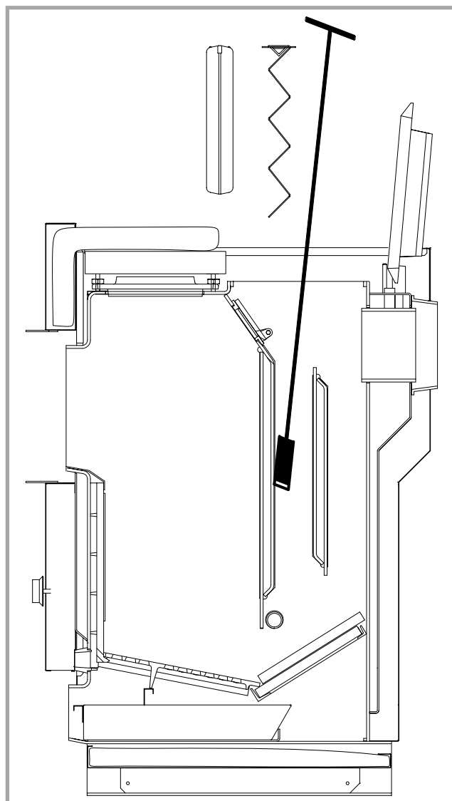
Figure 13 - Nettoyage de l'échangeur
