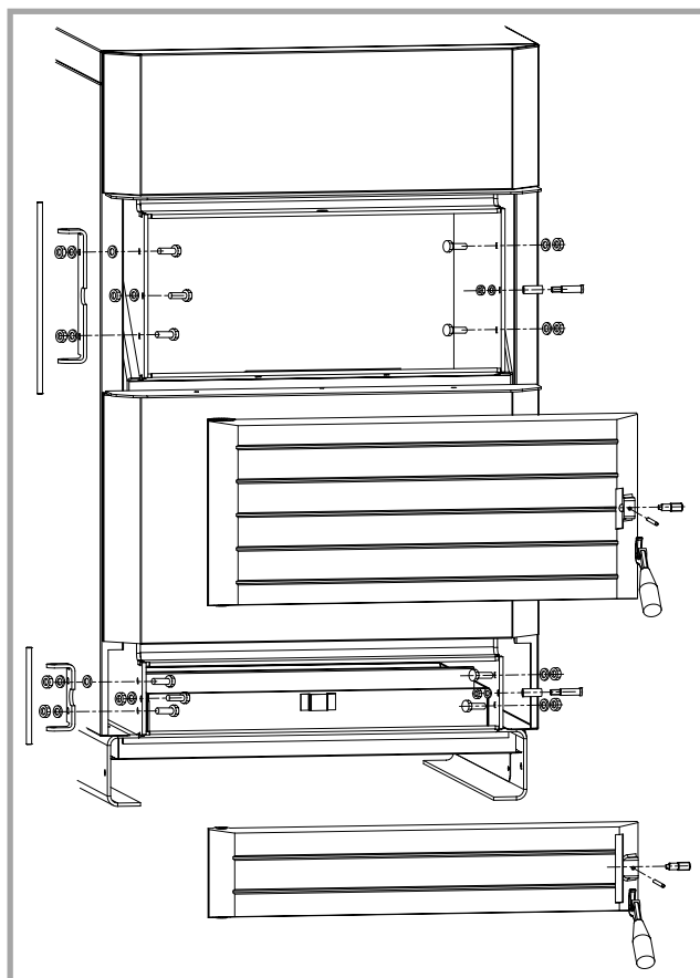
Figure 8 - Portes réversibles
