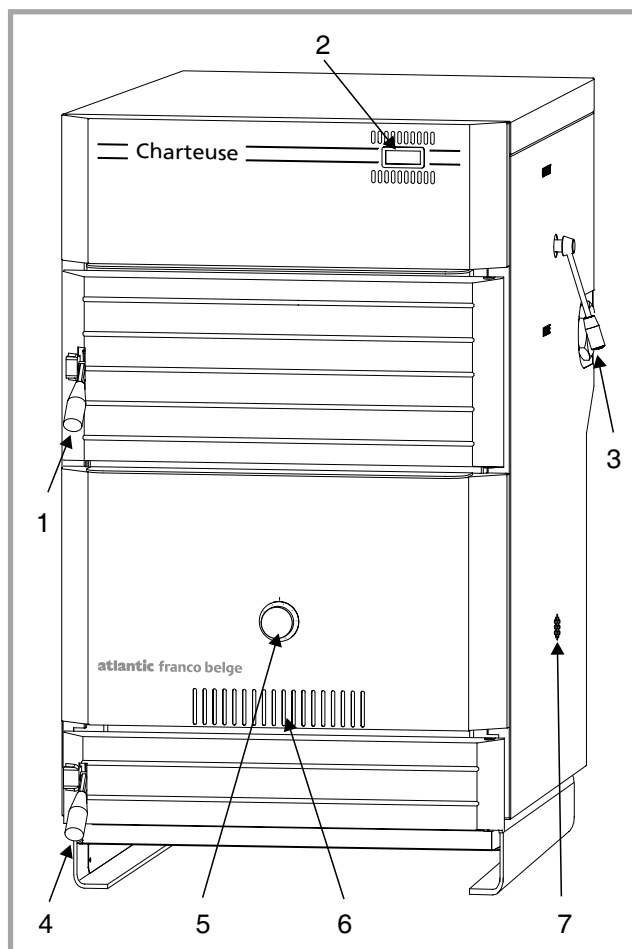
Figure 14 - Organes de commande et de contrôle
