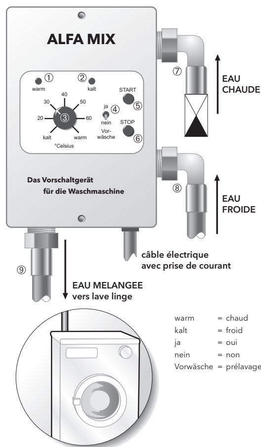
Fig. 1 Le prérelais thermique ALFA MIX pour raccorder une machine à laver un ballon d'eau chaude
