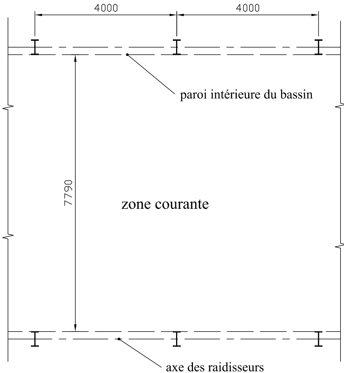
Plan partiel du bassin (vue de dessus)
