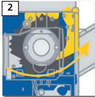
Fonction principale : les bouteilles sont percées par un rotor lent
