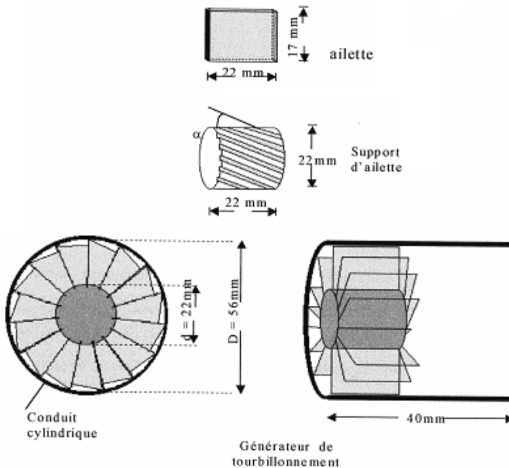
fig: Schéma du mode de génération de tourbillonnements
