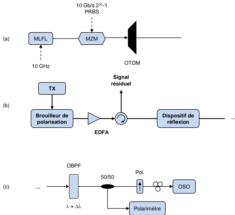
Figure 5.19 – Montage expérimental.
