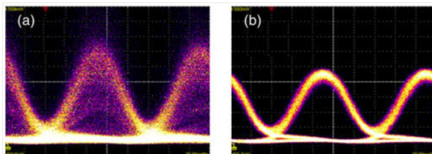
Figure 3.19 – Diagramme de l'œil du signal RZ à 10 Gb/s détecté derrière un polariseur : (a) en l'absence et (b) en présence de l'onde pompe.
