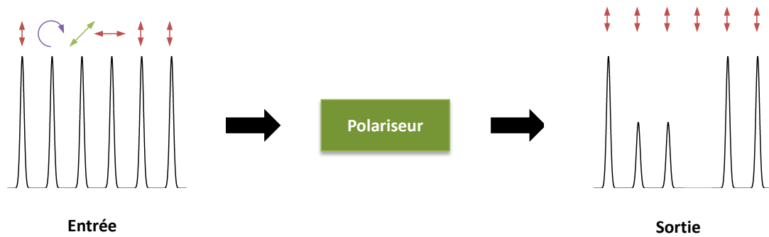
Figure 2.2 – Action d'un polariseur sur un train d'impulsions brouillé en polarisation.
