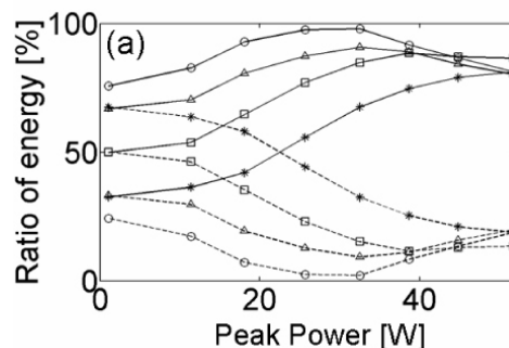
Figure 2.11 – Evolution de la quantité d'énergie du signal contenue dans les composantes circulaires droite (trait plein) et gauche (trait pointillé) pour différents états de polarisation du signal en fonction de la puissance des deux ondes (d'après [58]).
