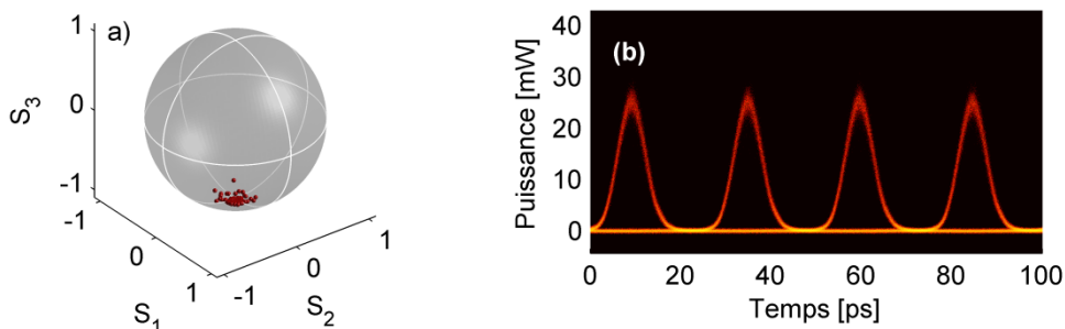
Figure 5.24 – A la sortie de l'omnipolariseur actif , (a) Etat de polarisation et (b) Diagramme de l'œil de l'onde signal RZ cadencé à 40 Gb/s en présence de l'onde signal réfléchie détectée après un polariseur et après modification de l'état de polarisation dans la boucle de réflexion amplifiée. Les puissances de l'onde signal et de l'onde signal réfléchie sont respectivement, de 500 mW et de 670 mW.
