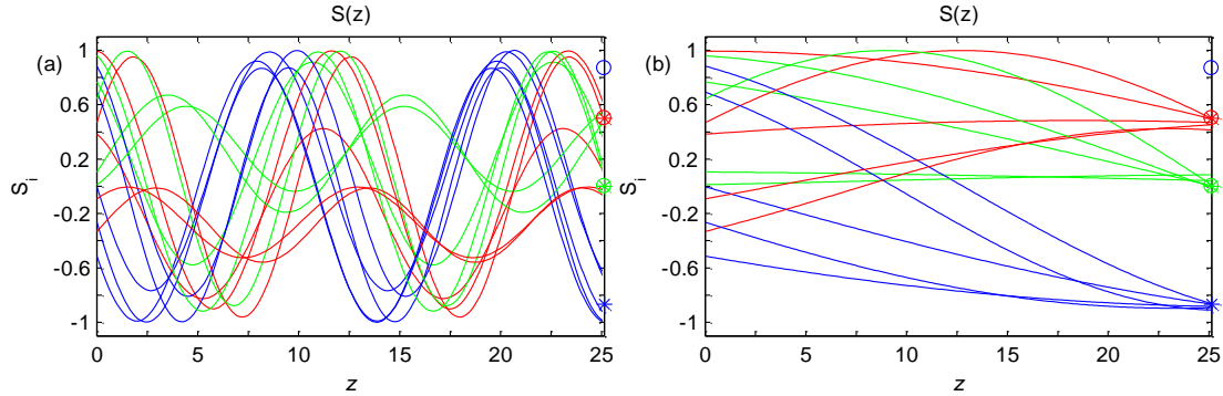
Figure 2.15 – Exemple de dépendance spatiale des paramètres de Stokes des solutions stationnaires (a) instables et (b) stables de l'onde signal ( S_1^+ , S_2^+ , S_3^+ ). S_1 : courbe bleue, S_2 : courbe verte et S_3 : courbe rouge. Les paramètres sont : L = 25 et S_0^+ = S_0^- .
