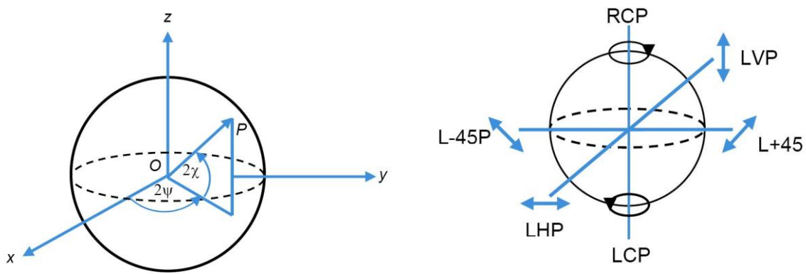
Figure 1.5 – (à gauche) Sphère de Poincaré et (à droite) Etats dégénérés de l'état de polarisation elliptique sur la sphère de Poincaré(d'après [18]).
