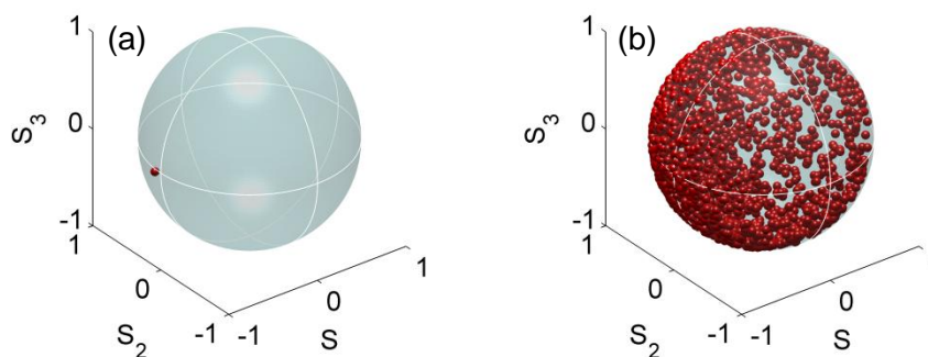
Figure 5.29 – Etat de polarisation de l'onde signal à la sortie de l'omni-polariseur actif (a) en l'absence et (b) en présence de l'onde signal réfléchie dans une fibre NZ-DSF de 6.2 km de long avec R = 10 .
