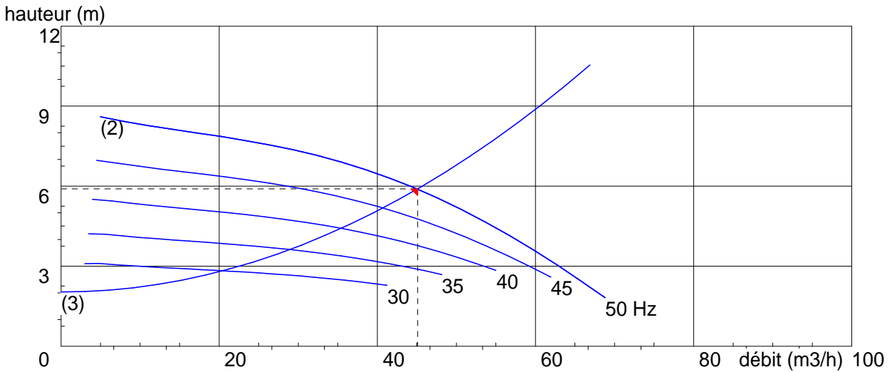
(1) Courbe individuelle (2) Courbe N Pompes (3) Courbe réseau
