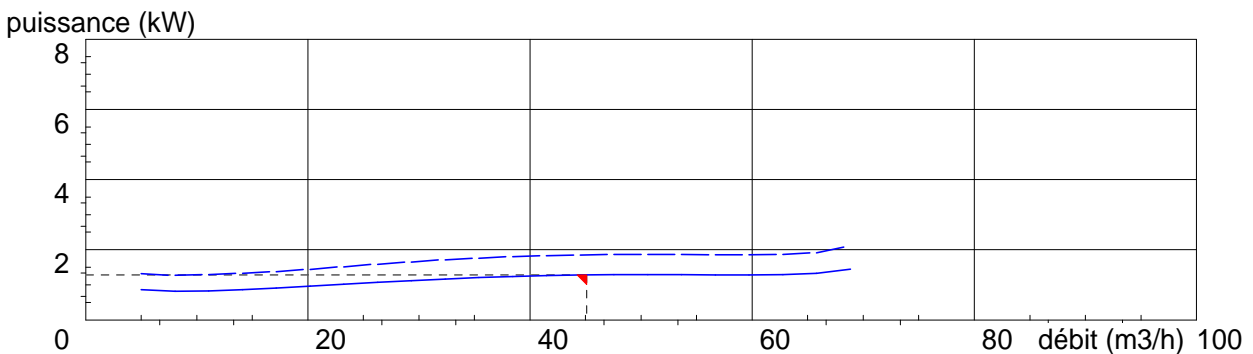
--- Puissance absorbée aux bornes ----- Puissance absorbée hydraulique
