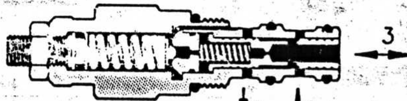
reduction 3 voies pilotée
