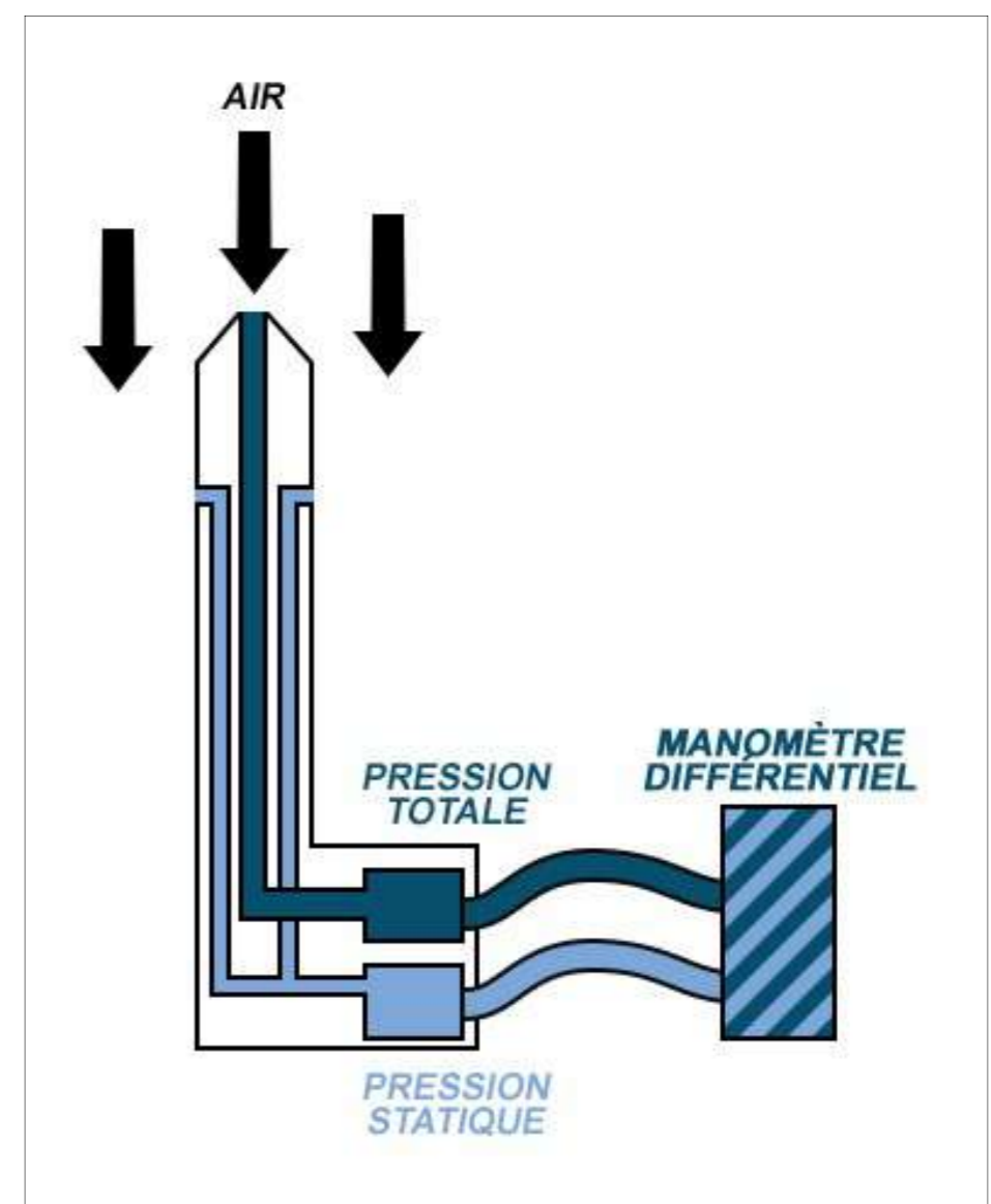
Schéma du tube de Pitot
