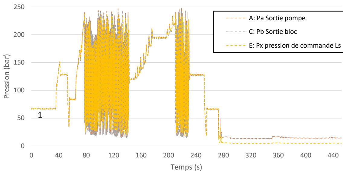
Variation des pressions Pa, Pb et Pc au cours de l'essai
